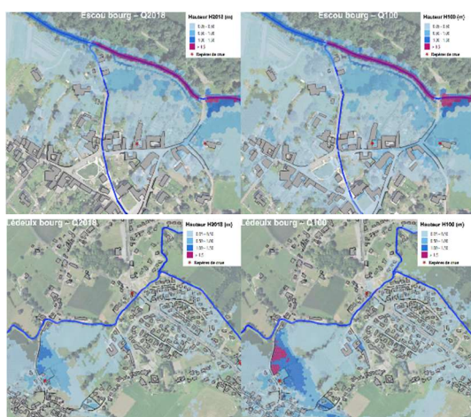
Modélisations hydrauliques pour Q_{2018} et Q_{100} – Source : HEA
